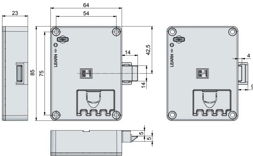
Lock M410 pro / Schloss M410 pro
