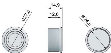
Fingerprint module / Fingermodul
